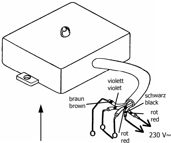
Anschlussbelegung und Stellung des eingebauten Relaiskontakts bei Tageslicht. Configuration of connections and position of the installed relay point at daylight.
