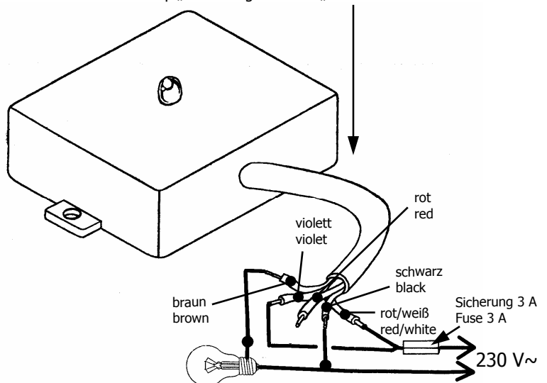
Anschluss: Lampe bei Dämmerungseintritt „EIN“ und bei Tagesanbruch „AUS“. Connection: Lamp „ON“ at nightfall and „OFF“ at dawn.
