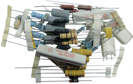
Hochlastwiderstände, verschiedene Typen
