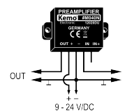
Anschluss für dynamische Mikrofone und andere Signalquellen
