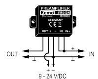
Anschluss für Elektretmikrofone
