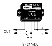
Anschluss für Elektretmikrofone
