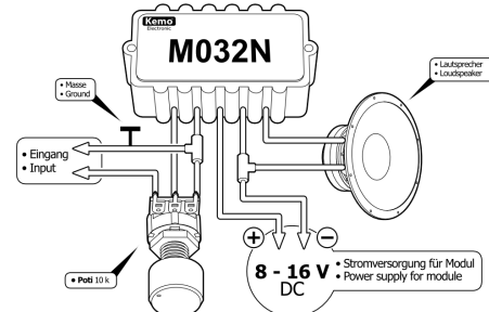
M032N
